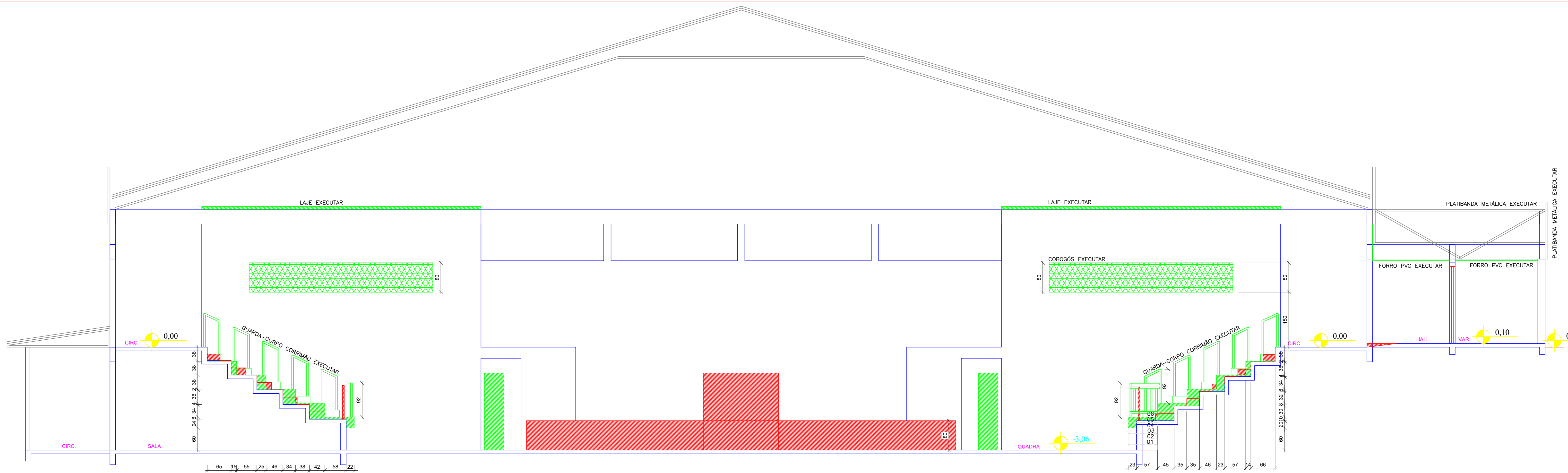
CORTE CC ESCALA 1:50
